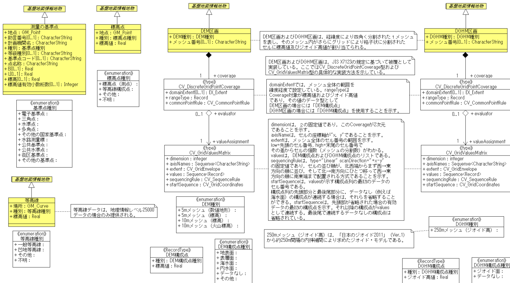
図 2-3 基準点等パッケージ
