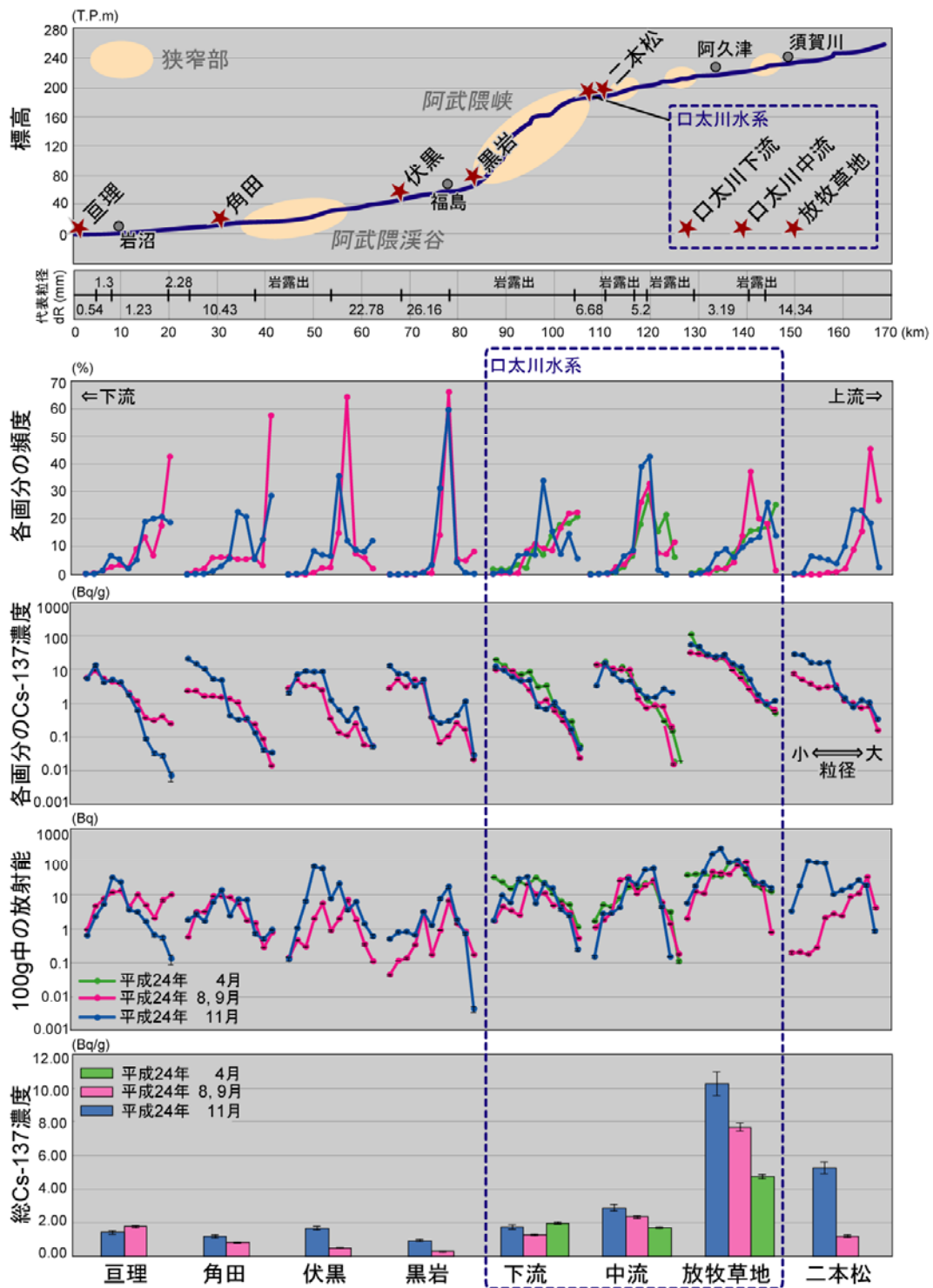
図 3.2.2(3)-3 阿武隈川の平均河床高縦断図（国交省、2004 [5]）及び河床の代表粒径と、各画分の頻度セシウム 137 濃度分布、堆積物 100 g 中のセシウム 137 の放射能、及び堆積物中の総セシウム 137 濃度（口太川下流及び放牧草地の試料は、第 2 次分布状況等調査報告書にて報告済み）
