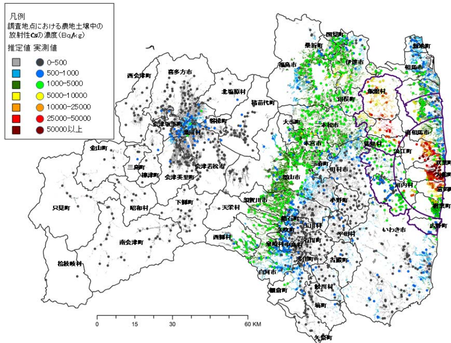
図 3.2.4(4)-7 福島県の農地土壌の放射性セシウム濃度の分布 (平成 23 年 11 月 5 日現在：農林水産省，2012)
