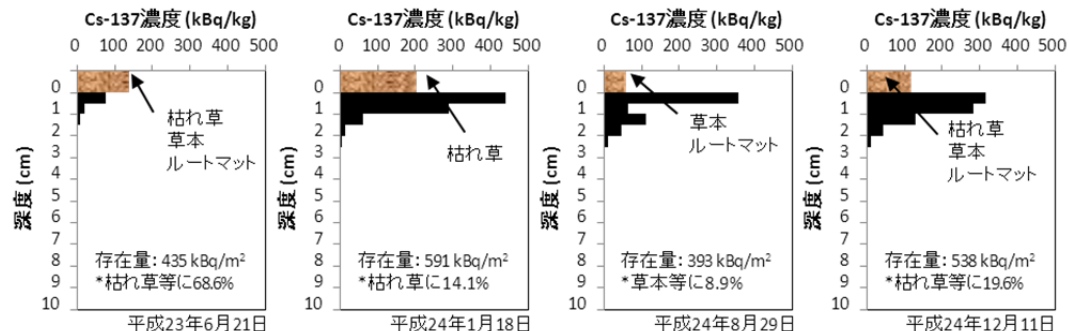
図 3.2.1(2)-1 各調査地点における土壌中のセシウム 137 の放射能濃度の深度分布及び単位面積あたりの放射性セシウム存在量の時間変化 (2) (左から第 1 回、第 2 回、第 3 回、第 4 回の調査結果を示し、枠外の日付は採取日を表す。 ※はリター量を補正した推定値。)
