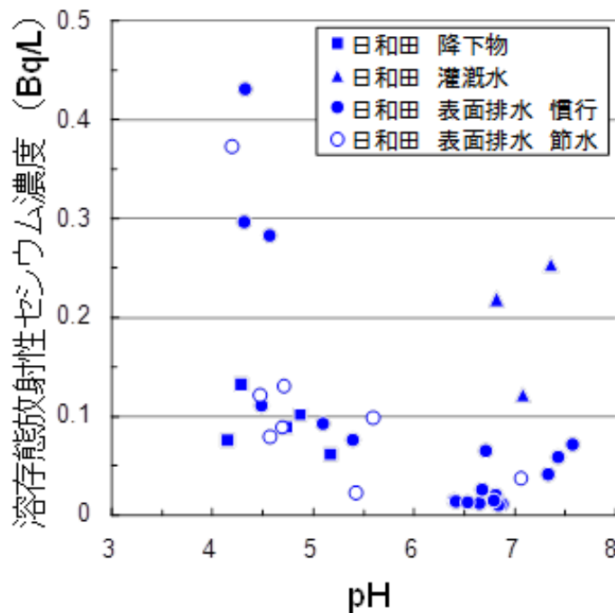
図 3. 2. 3-6 水試料中の pH と溶解放射能セシウム濃度の関係
