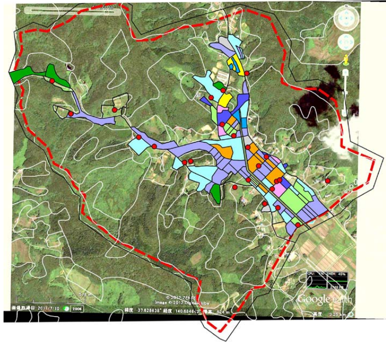
図 3. 2. 4(4)-9 飯館村比曾地区の植生分布図
