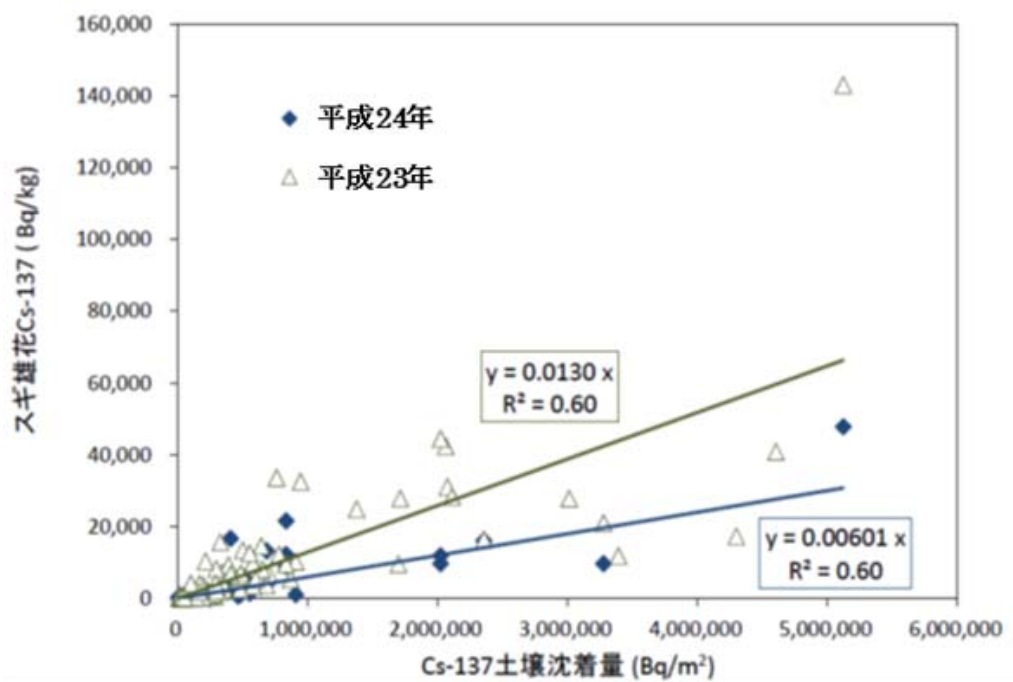
図 3.2.1(4)-4 土壌とスギ雄花のセシウム 137 濃度の関係 (平成 23 年及び平成 24 年)
