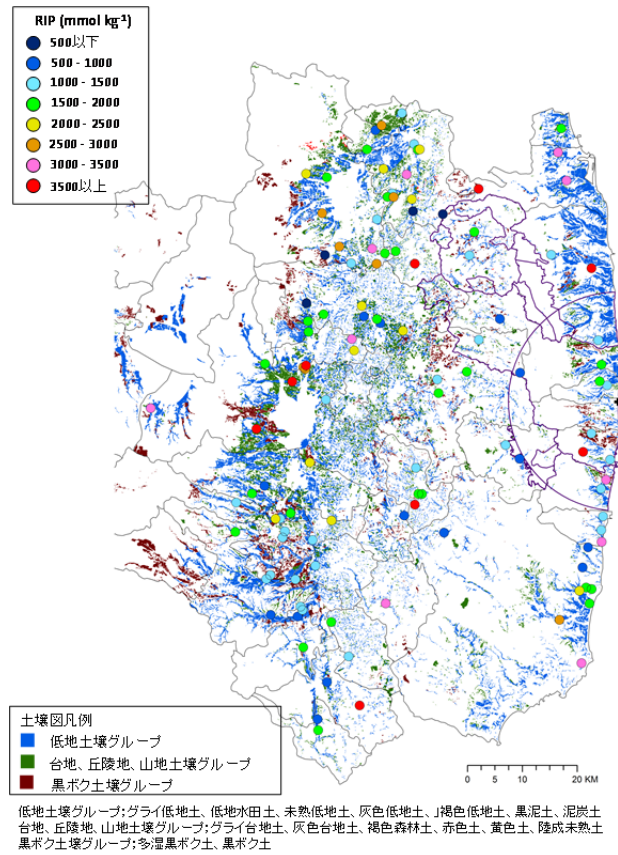
図 3. 2. 4(4)-10 福島第一原子力発電所から 80 km 圏内の農地土壤の RIP 値
