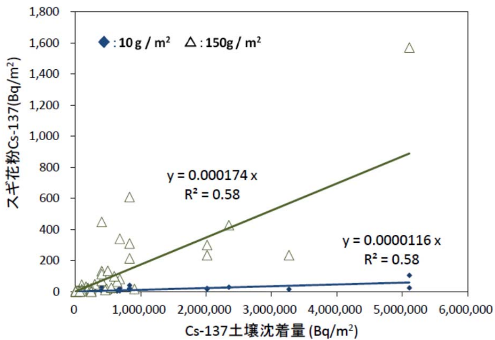
図 3. 2. 1(4)-6 異なるスギ雄花生産量において飛散する花粉中のセシウム 137 存在量と土壤への沈着量との関係
