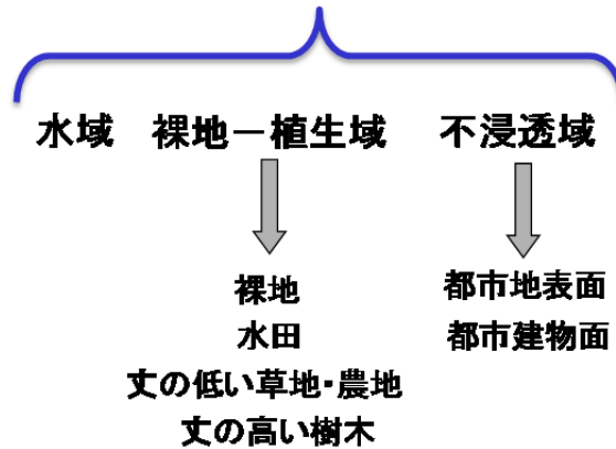
図 3. 2. 4(3)-2 土地利用の再分類
