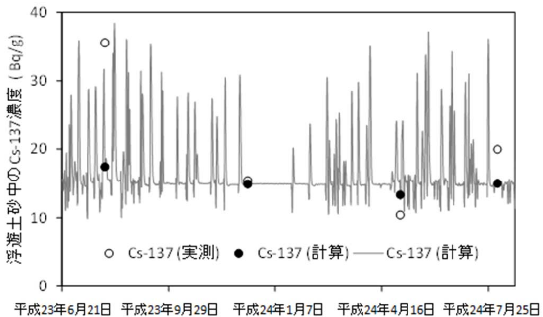
図 3.2.4(3)-6 セシウム 137 の濃度比較
