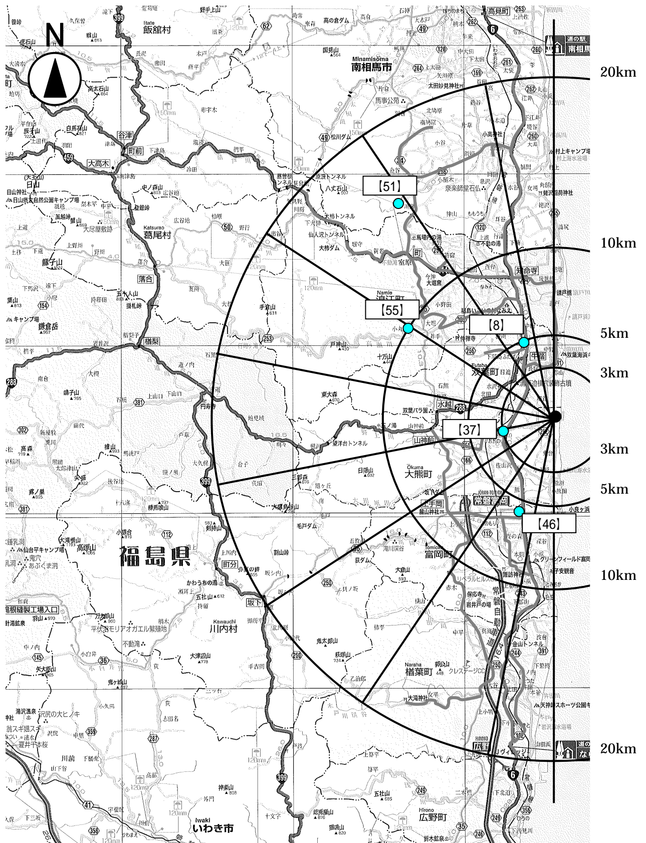
東京電力株式会社福島第一原子力発電所の20km圏内の土壤中放射性物質濃度測定を試料採取ポイント（採取日：平成24年10月16日）
