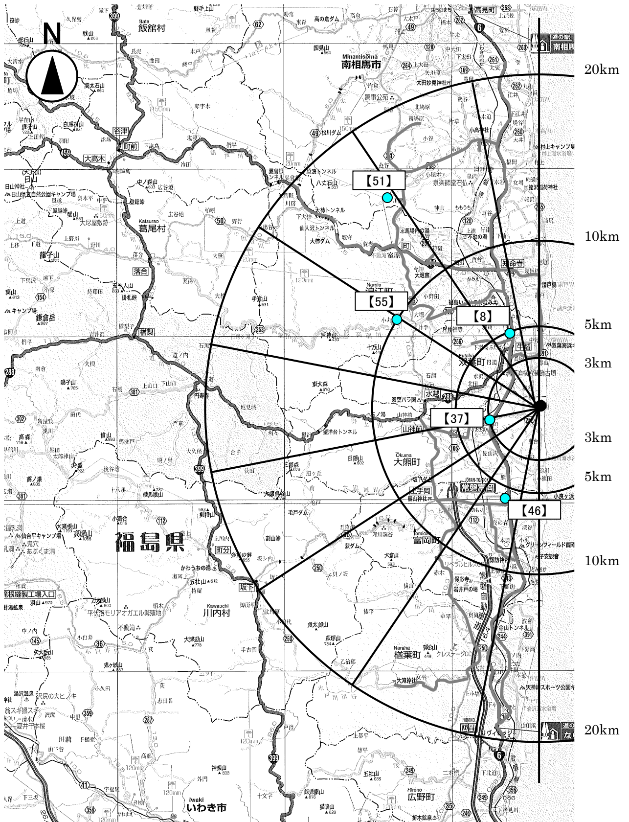
東京電力株式会社福島第一原子力発電所の20km圏内の土壤中放射性物質濃度測定のための試料採取ポイント（採取日：平成24年4月12日）
